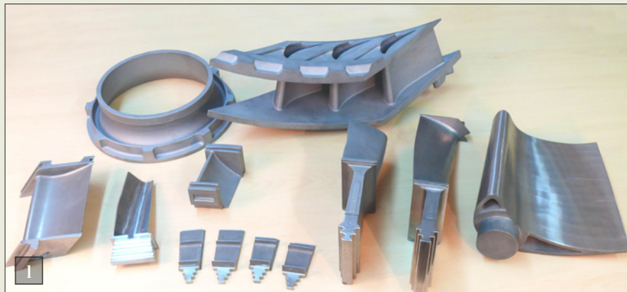
1. Продукция завода 2. Предварительный нагрев керамических форм
