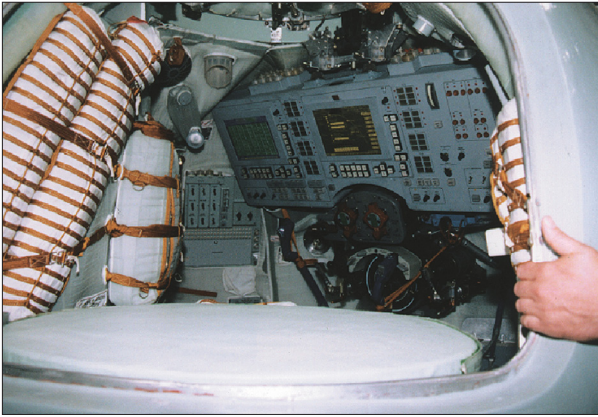
ДЕМОНСТРАЦИОННЫЙ МАКЕТ ПУЛЬТА КОСМОНАВТОВ
