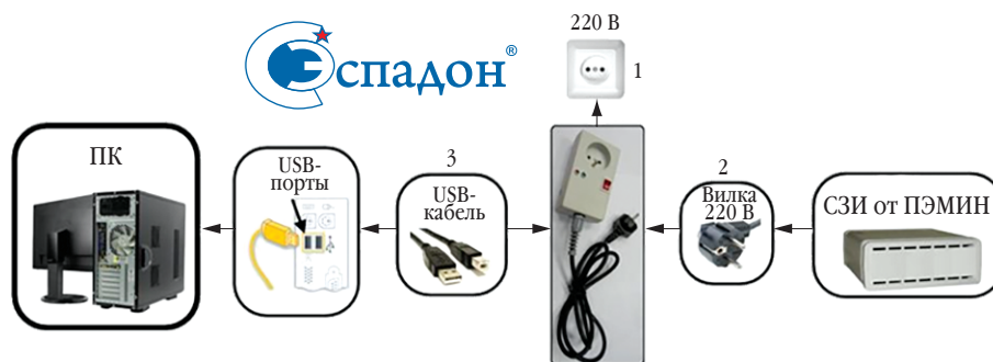
СХЕМА ПОДКЛЮЧЕНИЯ ИЗДЕЛИЯ КПУ-01
