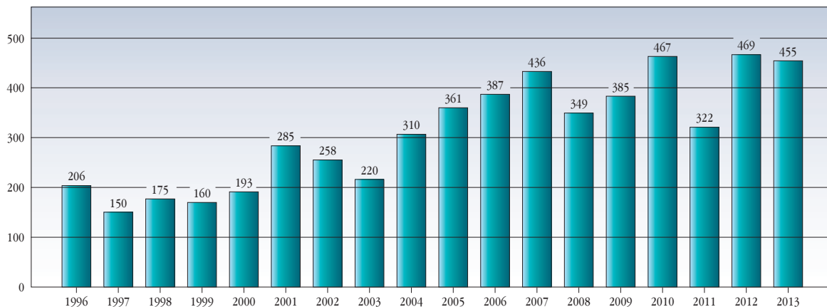
КОЛИЧЕСТВО ОПАСНЫХ ГИДРОМЕТЕОРОЛОГИЧЕСКИХ ЯВЛЕНИЙ В РОССИЙСКОЙ ФЕДЕРАЦИИ В 1996–2013 ГОДАХ, НАНЕСШИХ СЕРЬЕЗНЫЙ УЩЕРБ
